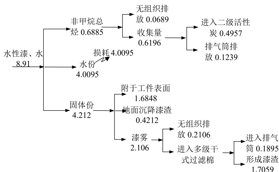
图 2-2 水性漆物料衡图 单位 t/a
