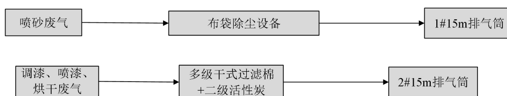
图 4-1 扩建项目废气处理工艺流程图
