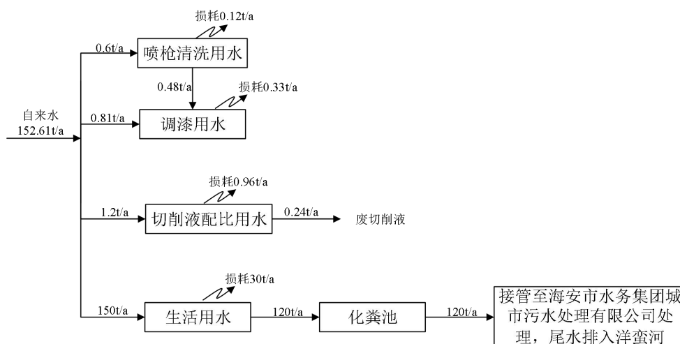
图 2-3 扩建项目水平衡图 单位 t/a
