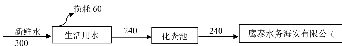
图 2-1 本项目用排水平衡图 (t/a)
